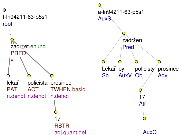
Obrázek 4.7: Dějová opisná pasivní diateze s aktorem a s pacientem v akuzativu (zadržet): Lékař byl zadržen policisty 17. prosince
