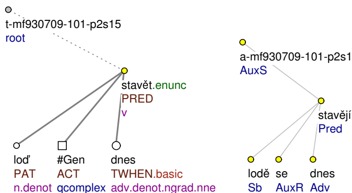
Obrázek 4.17: Pasivní reflexivní diateze s aktorem a patientem v akuzativu v rámci (stavěť): lodě se dnes stavějí ...
