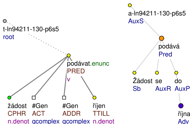
Obrázek 4.23: Pasivní reflexivní diateze s funktorem CPHR ( podávat žádost ): Žádost se podává do října
