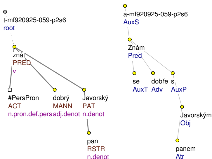
Obrázek 4.34: Reciproční užití slovesa znát v PDT: Znám se dobře s panem Javorským
