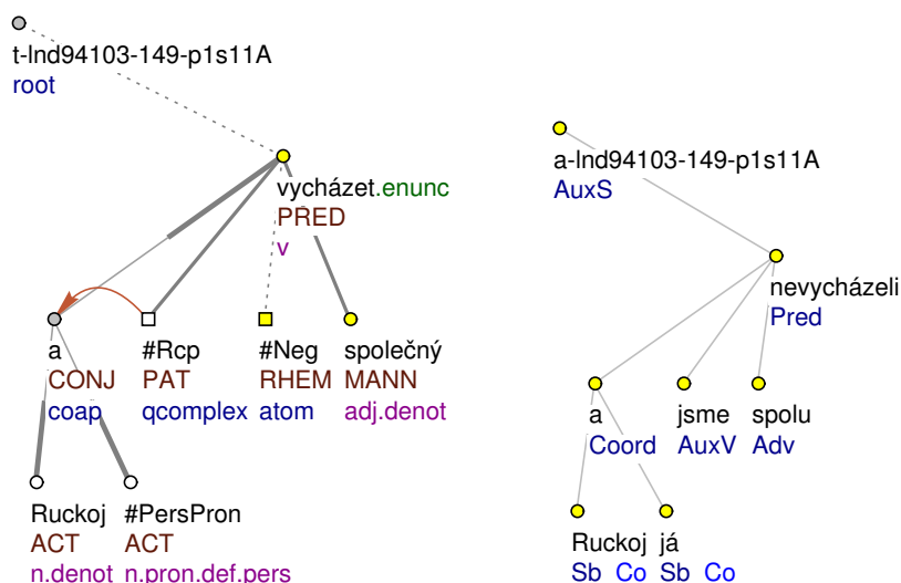
Obrázek 4.32: Reciproční vztah mezi ACT a PAT, sloveso vycházet : Ruckoj a já jsme spolu nevycházeli
