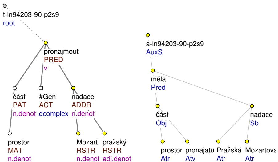
Obrázek 4.26: Tektogrammatická a analytická reprezentace se slovesem pronajmout : ...měla část prostor pronajatu Pražská Mozartova nadace
