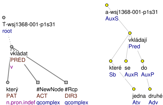
Obrázek 4.44: Syntaktické vyjádření reciprocity, podtyp 5, akuzativ (po reflexivní pasivizaci nominativ) a předložka do s genitivem, sloveso vkládat : ..., které se vkládají jedna do druhé (příklad z překladu PTB III, část WSJ)
