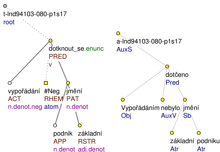
Obrázek 4.14: Anotace opisného pasiva se slovesem dotknout se : Vypořádáním nebylo dotčeno základní jmění podniku
