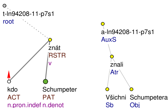
Obrázek 4.33: Nereciproční užití slovesa znát v PDT: Všichni znali Schumpetera
