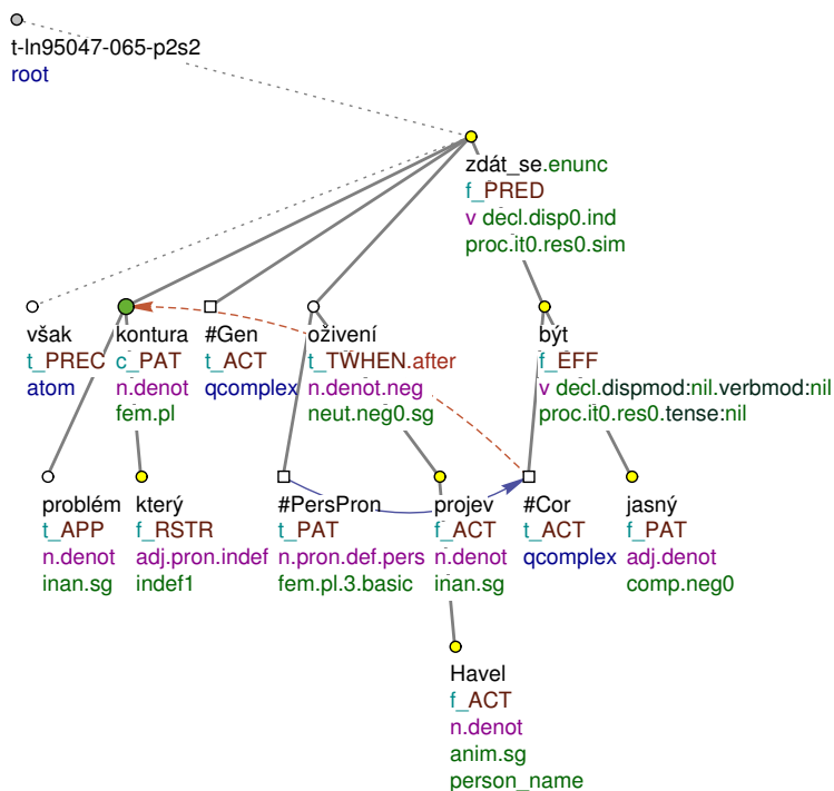
Obrázek 3.1: Ukázka tektogramatické anotace v PDT: Některé kontury problému se však po oživení Havlovým projevem zdají být jasnější.
