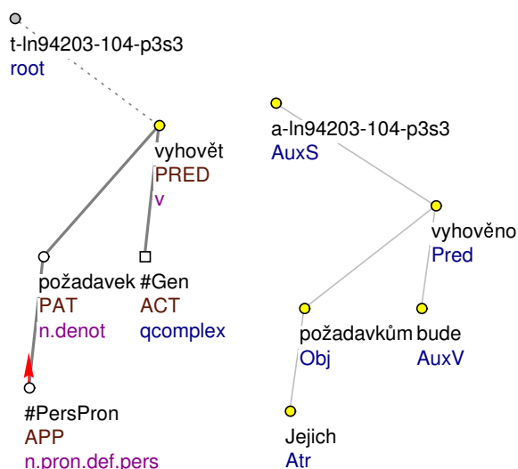
Obrázek 4.6: Dějová opisná pasivní diateze s pacientem v dativu ( vyhovět ): Jejich požadavkům bylo vyhověno
