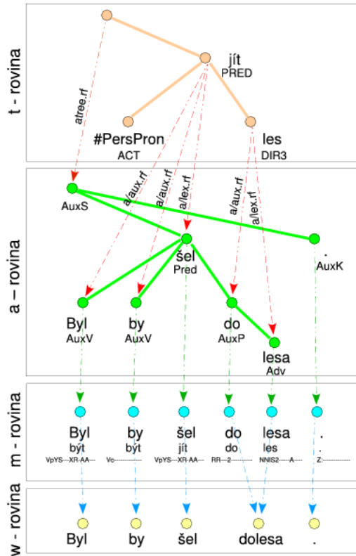
Obrázek 3.3: Propojení rovin anotace v PDT
