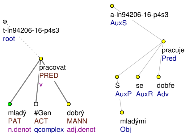
Obrázek 4.30: Dispoziční modalita ( pracovat )
