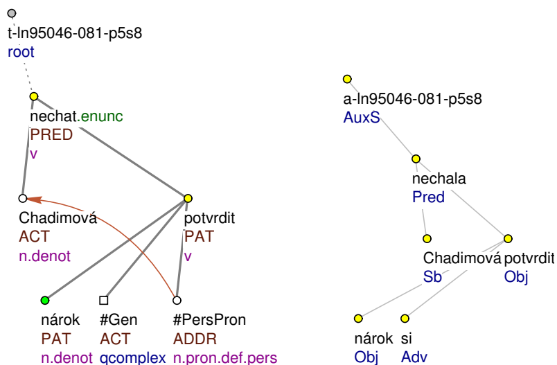
Obrázek 4.31: Tektogramatická a analytická reprezentace kauzativní konstrukce se slovesem nechat : ...nárok si nechala Chadimová potvrdit
