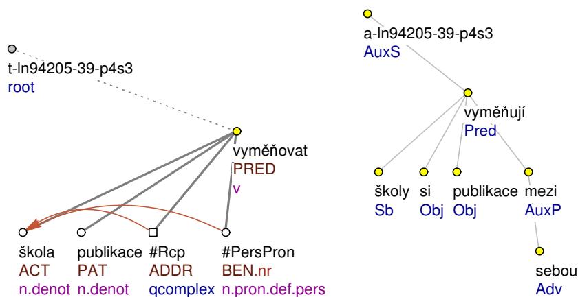
Obrázek 4.42: Syntaktické vyjádření reciprocity, podtyp 3 (nominativ – s+instrumentál), sloveso vyměňovat : školy si publikace vyměňují mezi sebou
