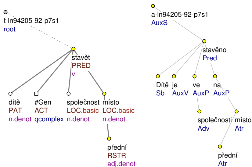
Obrázek 4.3: Tektogramatická a analytická reprezentace děje (opisné pasivum): Dítě je ve společnosti stavěno na první místo
