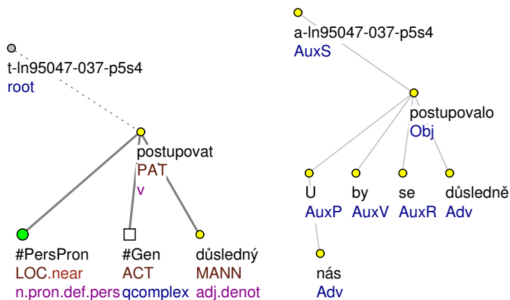
Obrázek 4.15: Pasivní reflexivní diateze s jediným aktantem v rámci ( postupovat ): U nás by se postupovalo důsledně
