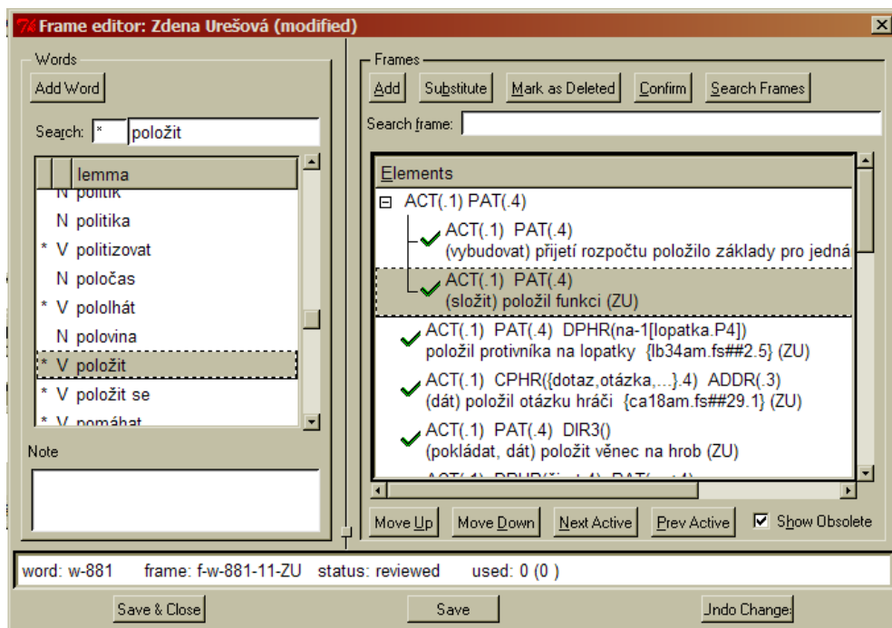
Obrázek 3.7: Uživatelské rozhraní slovníku PDT-Vallex v TrEdu
