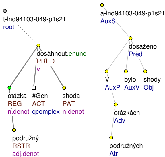
Obrázek 4.8: Dějová opisná pasivní díateze s patientem v genitivu (na povrchu zachovaným, dosáhnout ): V podružných otázkách bylo dosaženo shody.
