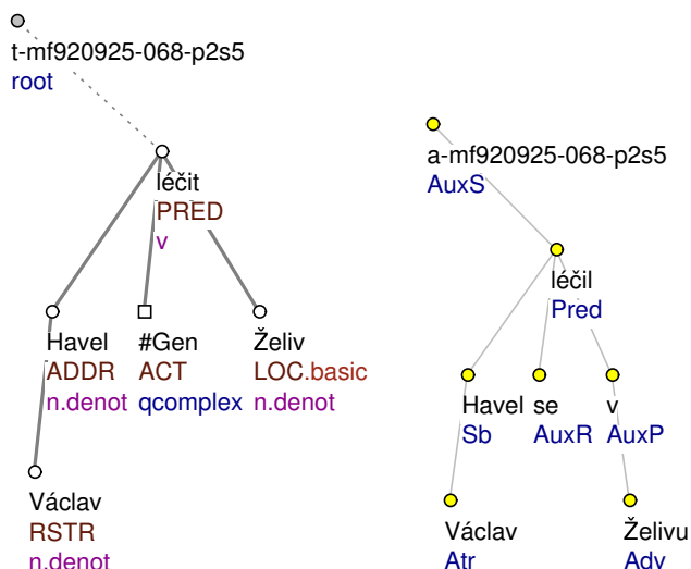
Obrázek 4.20: Pasivní reflexivní diateze, adresát v akuzativu, sloveso léčit : Václav Havel se léčil v Želivu
