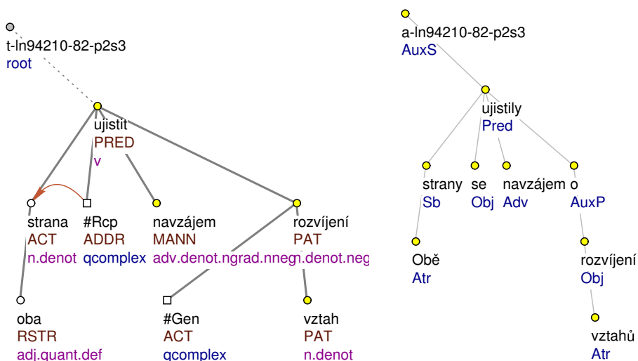
Obrázek 4.39: Syntakticky vyjádřená reciprocita, podtyp 1 (nominativ – akuzativ), sloveso ujistit : Obě strany se ujistily navzájem o rozvíjení vztahů
