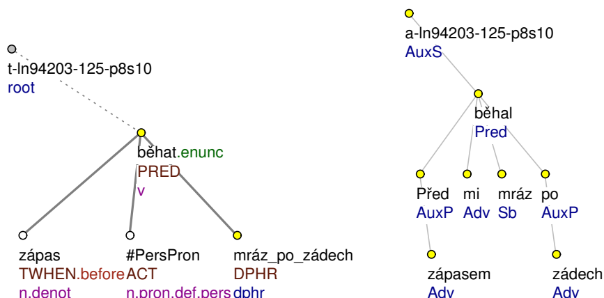
Obrázek 3.6: Anotace frazeologického spojení: Před zápasem mi běhal mráz po zádech
