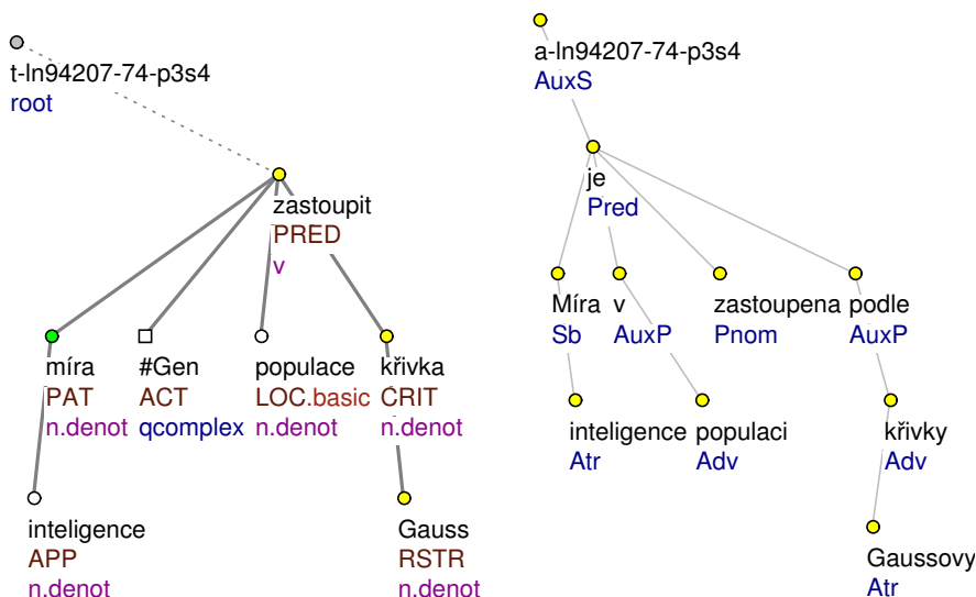
Obrázek 4.29: Tektogrammatická a analytická reprezentace stavu se slovesem zastoupit : Míra inteligence je v populaci zastoupena podle Gaussovy křivky
