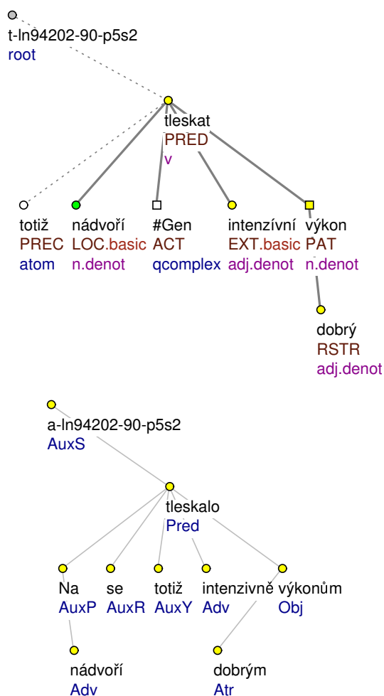
Obrázek 4.16: Pasivní reflexivní diateze s pacientem v dativu ( tleskat ): Na nádvoří se totiž tleskalo intenzivně dobrým výkonům
