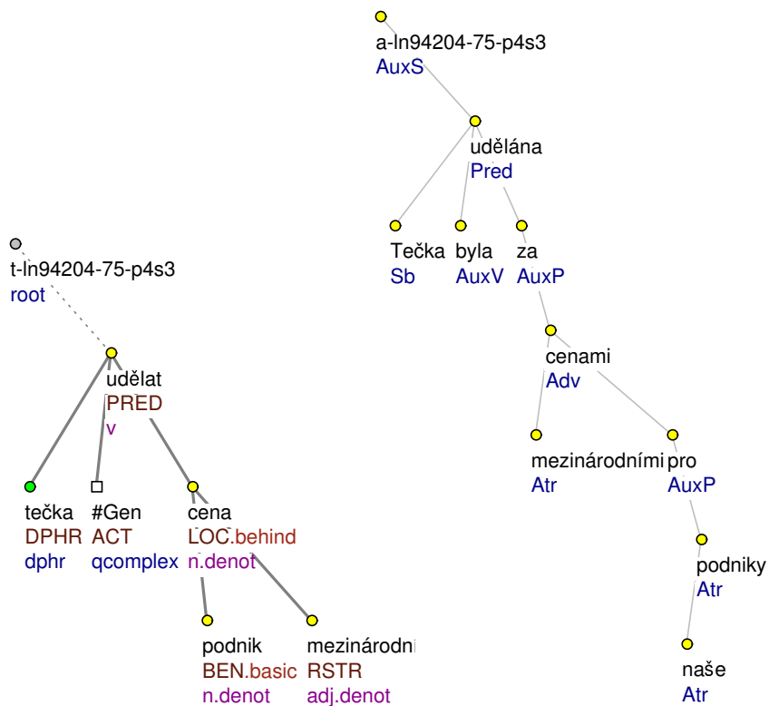
Obrázek 4.12: Dějová opisná pasivní diateze s funktorem DPHR (udělat tečku): Tečka byla udělána za mezinárodními cenami pro naše podniky
