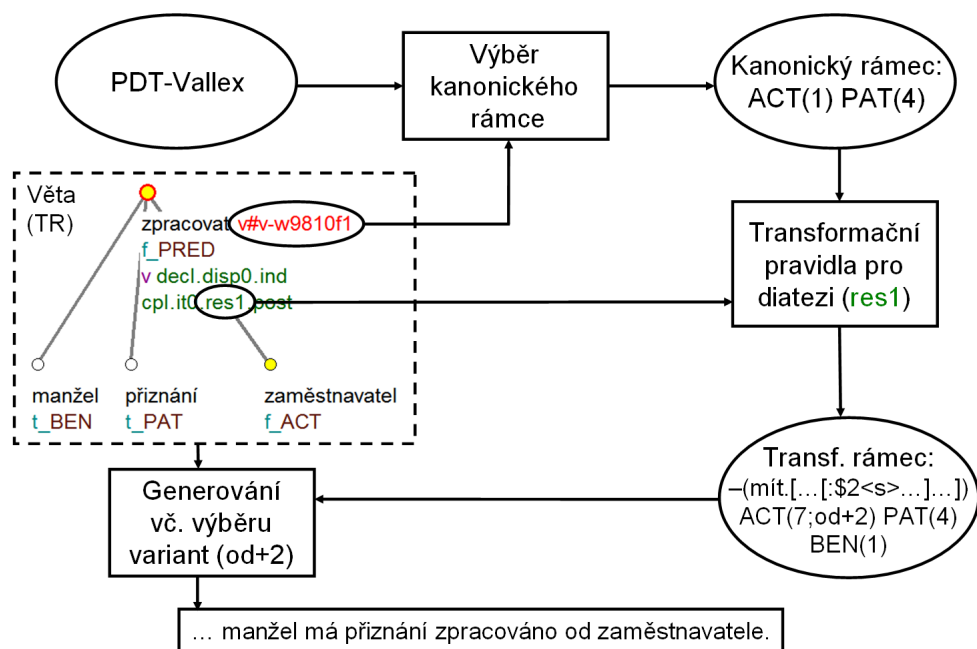
Obrázek 4.1: Možné schéma aplikace transformačních pravidel užitých při aplikaci na generování vět
