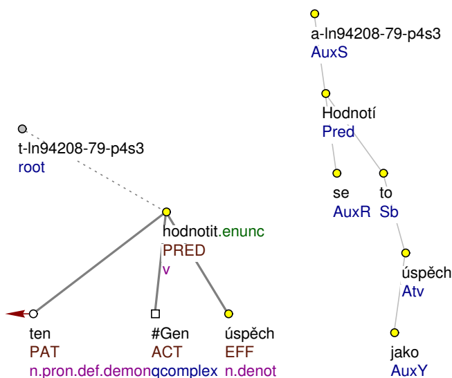
Obrázek 4.19: Pasivní reflexivní diateze s aktorem a pacientem v akuzativu a efektem s vazbou jako s akuzativem ( hodnotit ): Hodnotí se to jako úspěch .
