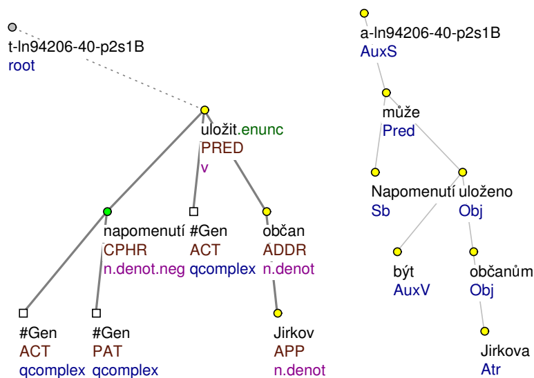
Obrázek 4.13: Dějová opisná pasivní diateze s funktorem CPHR ( uložit napomenutí ): Napomenutí může být uloženo občany Jirkova
