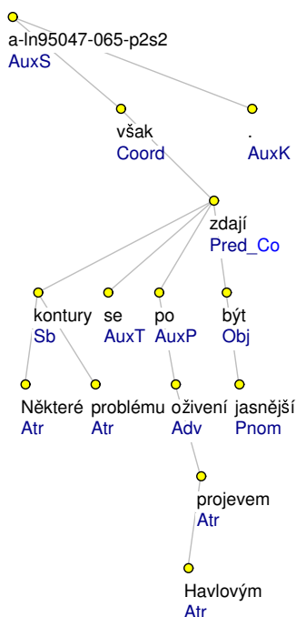
Obrázek 3.2: Ukázka analytické anotace v PDT (stejná věta jako na obr. 3.1)
