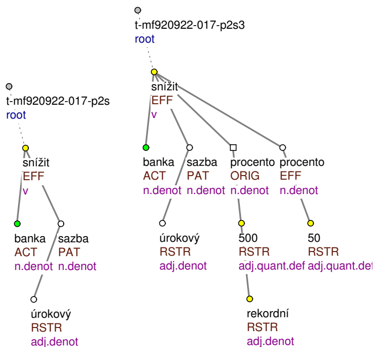
Obrázek 3.8: Postupné „přibývání“ fakultativních aktantů u slovesa snížit
