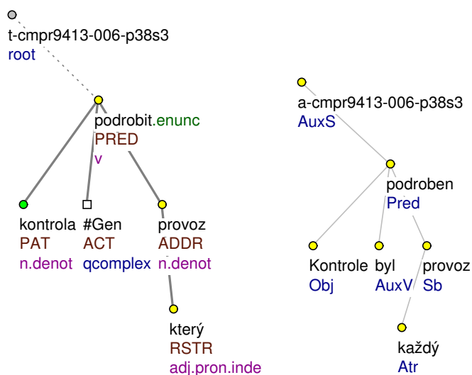
Obrázek 4.10: Dějová opisná pasivní diateze s adresátem v akuzativu ( podrobit ): Kontrola byl podroben každý provoz
