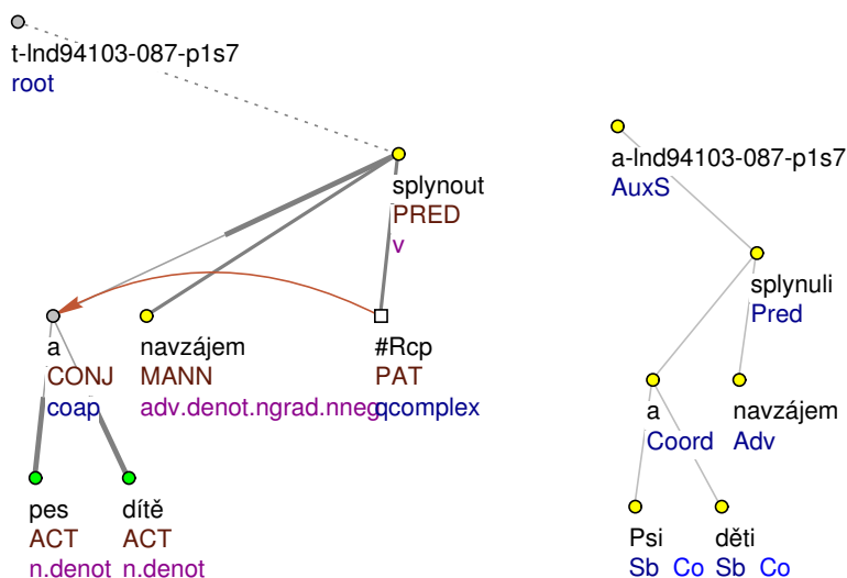
Obrázek 4.41: Syntaktické vyjádření reciprocity, podtyp 3 (nominativ – s+instrumentál), sloveso splynout : Psi a děti navzájem splynuli
