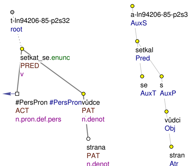
Obrázek 4.36: Inherentní reciproční vztah mezi aktorem a pacientem: setkal se s vůdci stran
