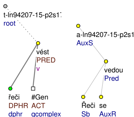
Obrázek 4.22: Pasivní reflexivní diateze s funktorem DPHR ( vést řeči ): Řeči se vedou
