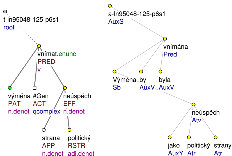
Obrázek 4.9: Dějová opisná pasivní diateze s pacientem v akuzativu a efektem s vazbou jako s akuzativem ( vnímat ): Výměna by byla vnímána jako politický neúspěch strany
