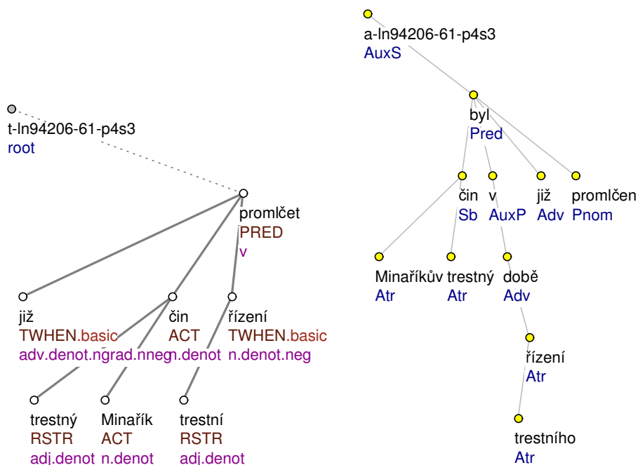
Obrázek 4.28: Tektogrammatická a analytická reprezentace stavu se slovesem promlčet : Minaříkův trestný čin byl v době trestního řízení již promlčen
