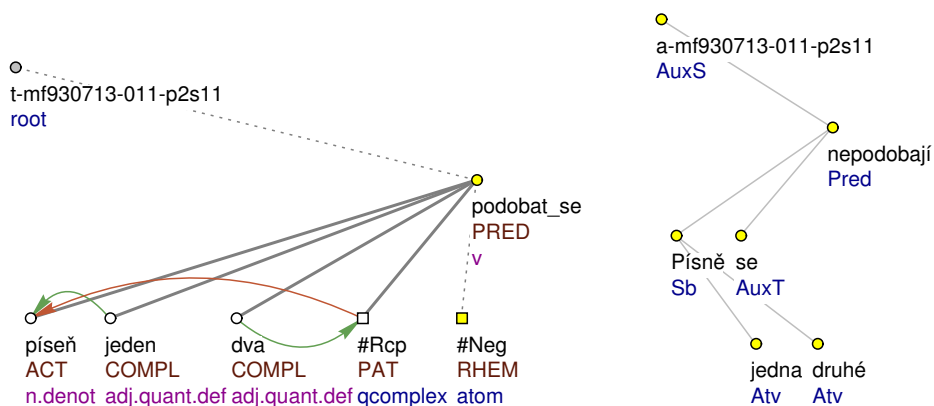
Obrázek 4.40: Syntakticky vyjádřená reciprocita, podtyp 2 (nominativ – dativ), sloveso podobat se : Písně se jedna druhé nepodobají
