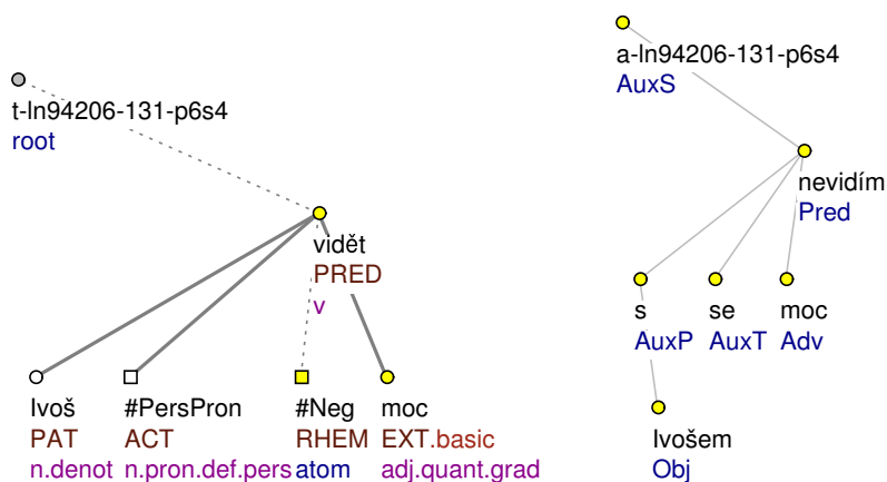
Obrázek 4.37: Zachycení recipročního užití slovesa vidět v textogramatické a analytické anotaci: s Ivošem se moc nevidím
