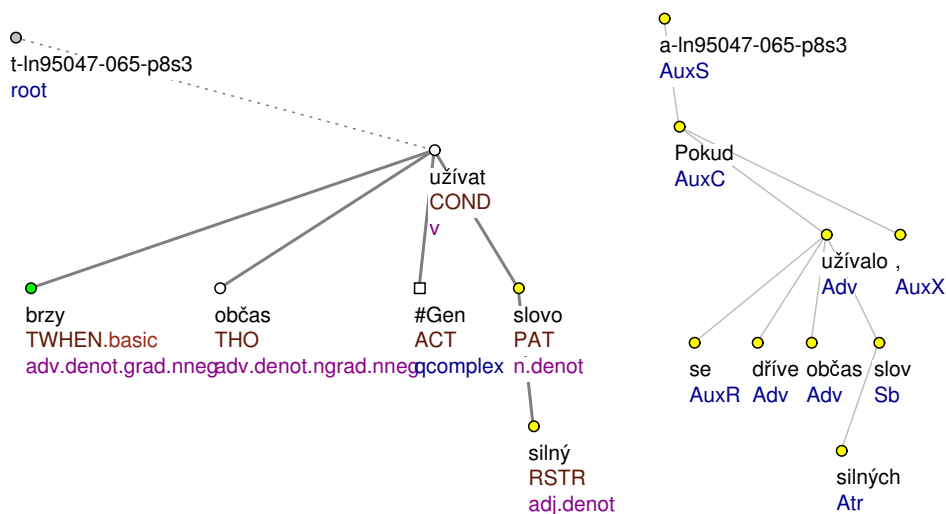
Obrázek 4.18: Pasivní reflexivní diateze s aktorem a pacientem v genitivu ( užívat ): Pokud se dříve užívalo silných slov, ...
