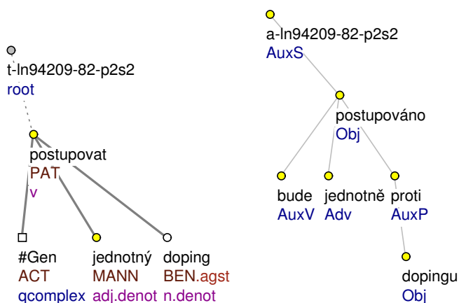
Obrázek 4.5: Dějová opisná pasivní diateze s jediným aktantem v rámci ( postupovat ): ...bude jednotně postupováno proti dopingu
