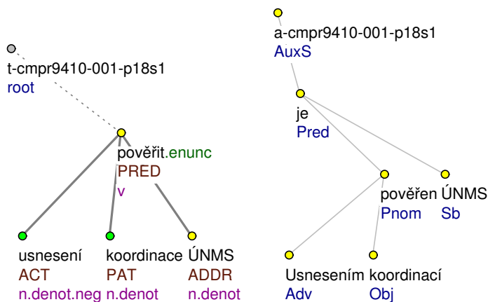
Obrázek 4.4: Tektogramatická a analytická reprezentace stavu (rezultativ s být ): Usnesením je koordinací pověřen ÚNMS
