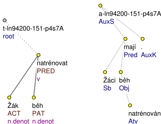
Obrázek 4.25: Rezultativ se slovesem mít , sloveso natrénovat : Žáci mají běh natrénován
