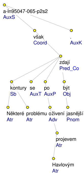
Obrázek 4.2: Ukázka analytické anotace v PDT (stejná věta jako na obr. 4.1)
