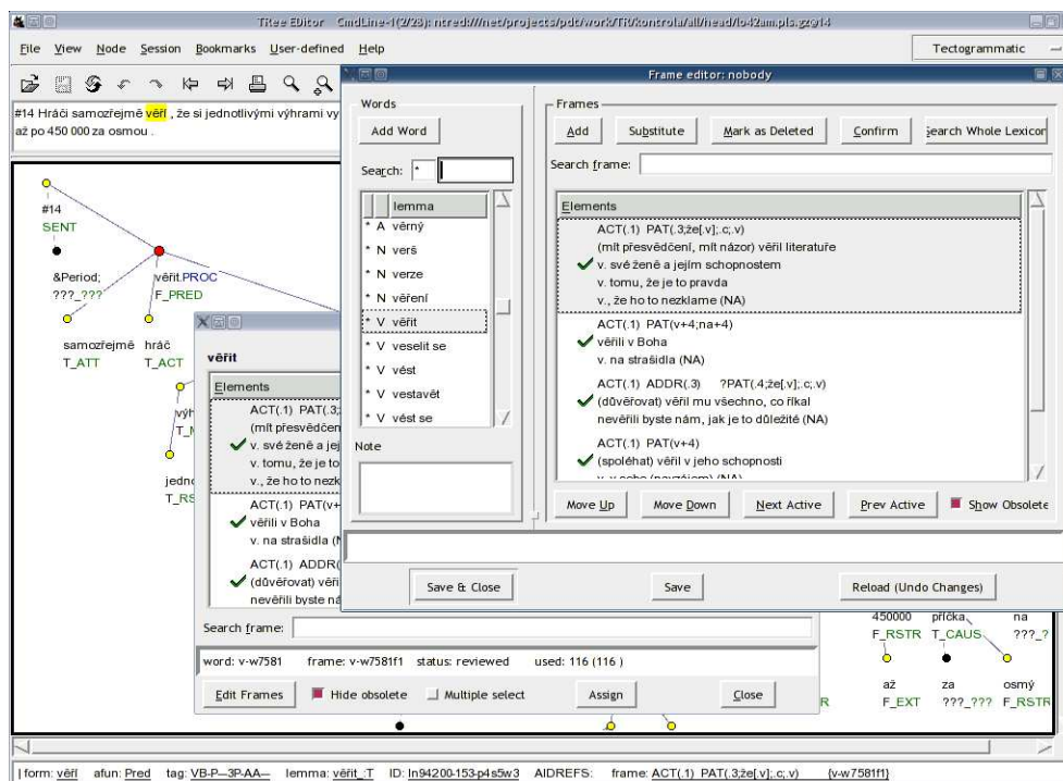
Obrázek 4.7: Uživatelské rozhraní slovníku PDT-Vallex v TrEdu
